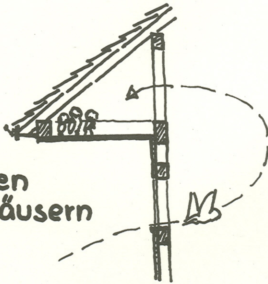
Schnitt A-A
